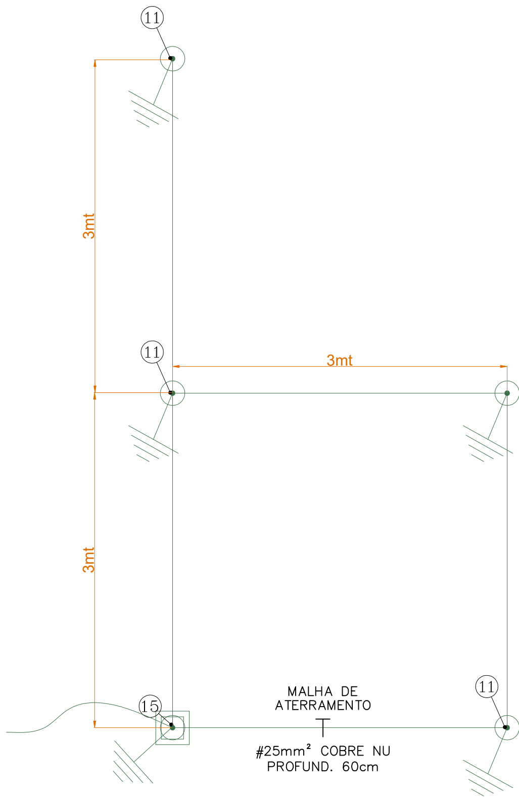
DETALHE ATERRAMENTO SEM ESCALA
