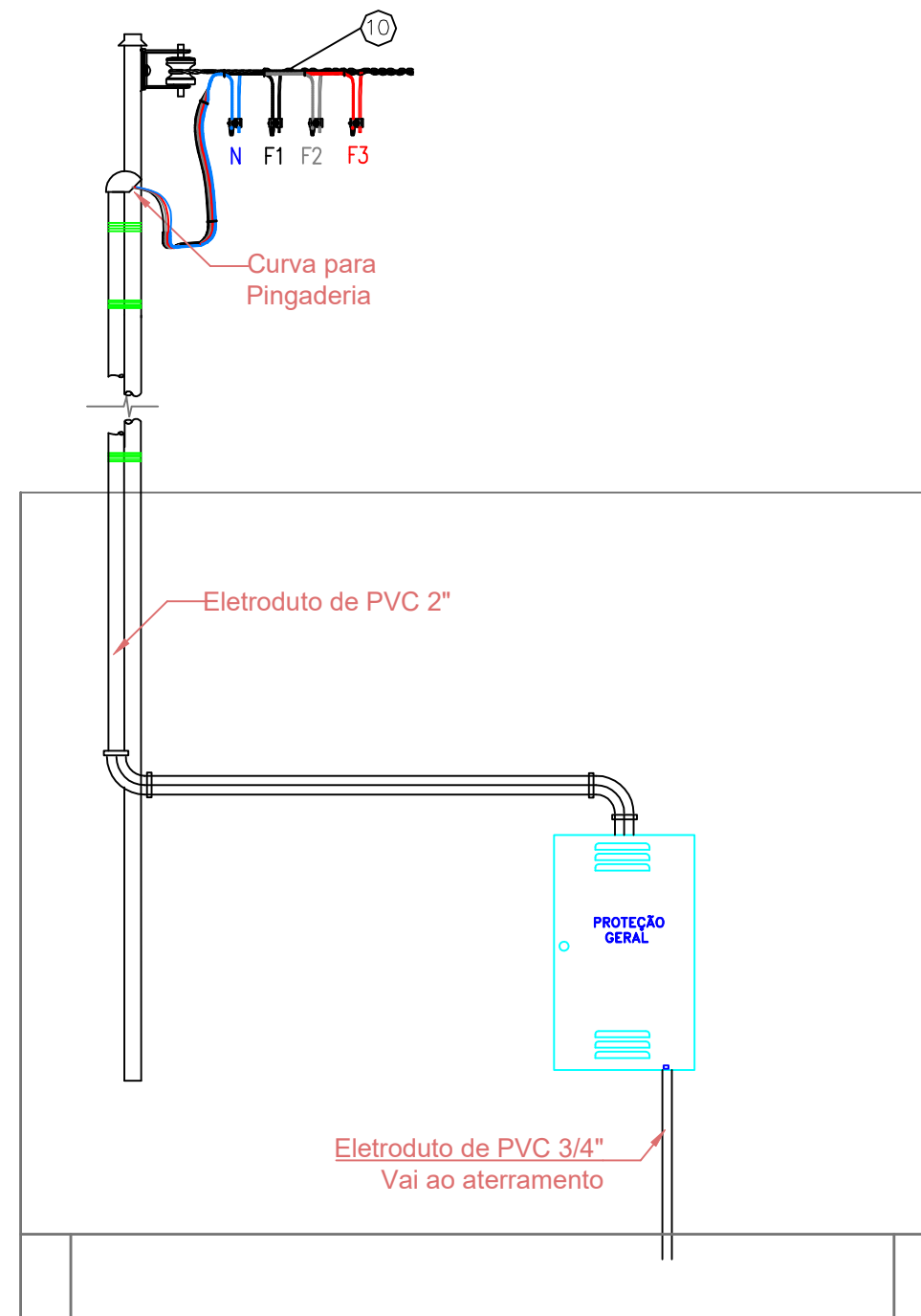
DETALHE PONTALETE SEM ESCALA
