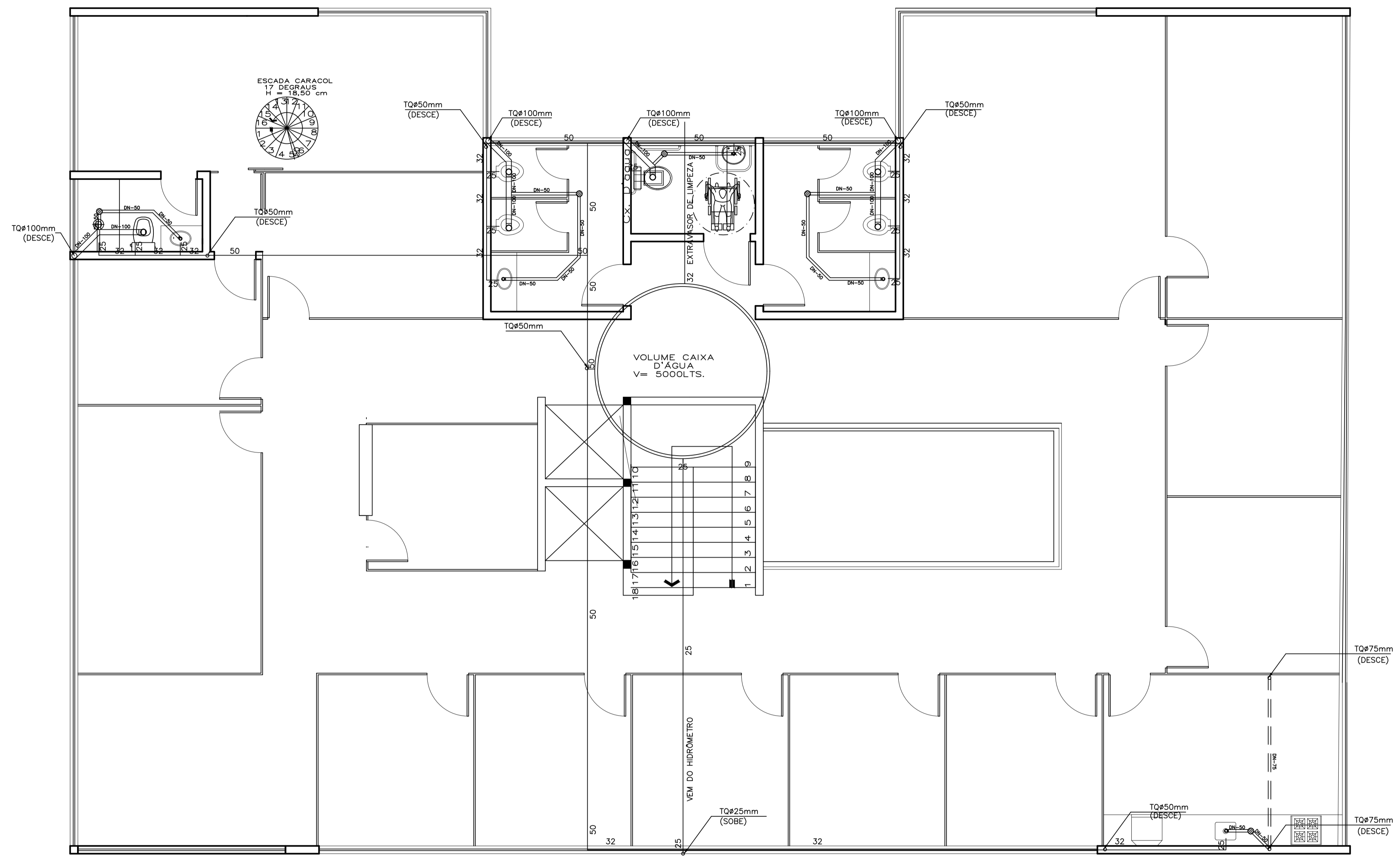
PAVÃO SUPERIOR HIDROSSANITÁRIO ESCALA 1/50
