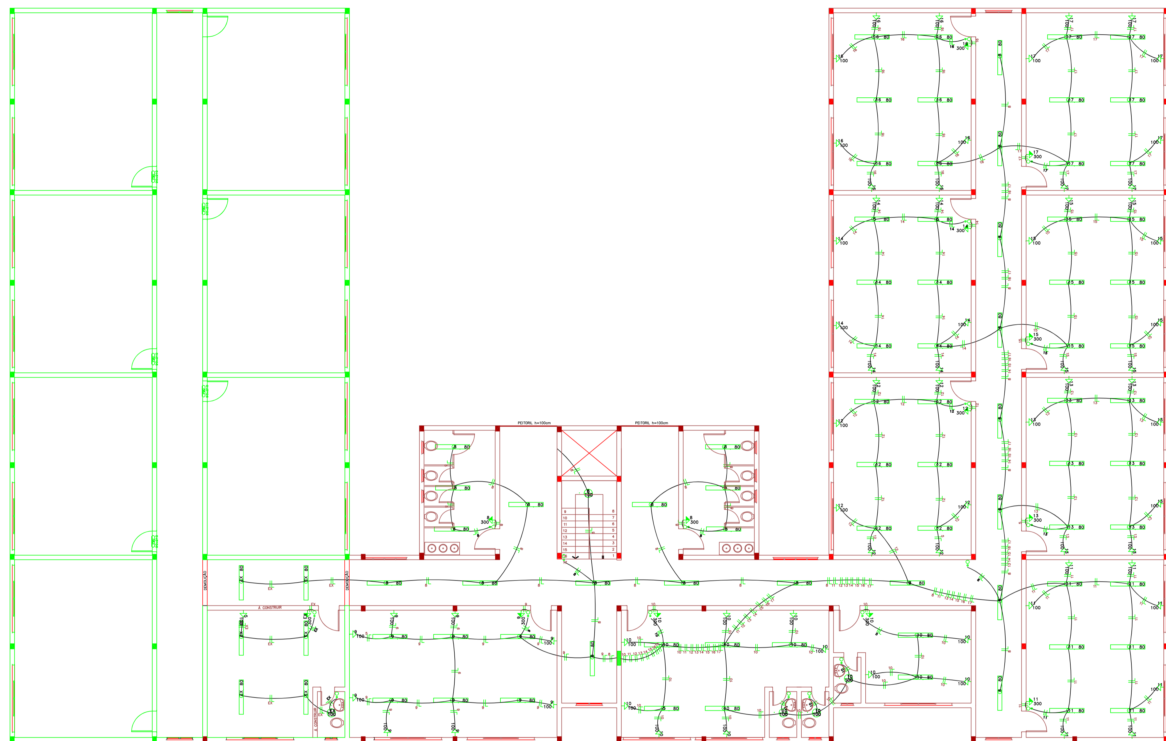
PAVTO SUPERIOR ELÉTRICO ESC: 1/50
