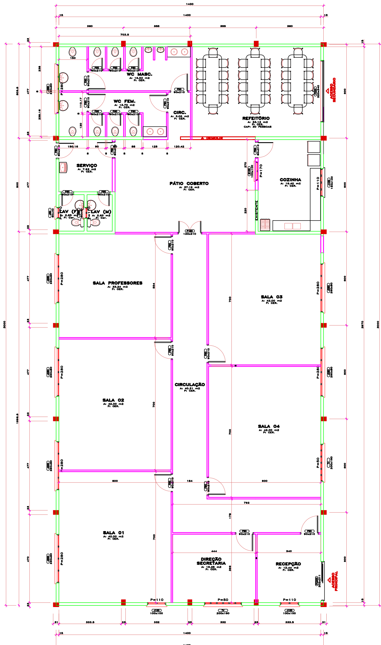
PLANTA BAIXA Escola 1/75 Ai 429,00 m 2
