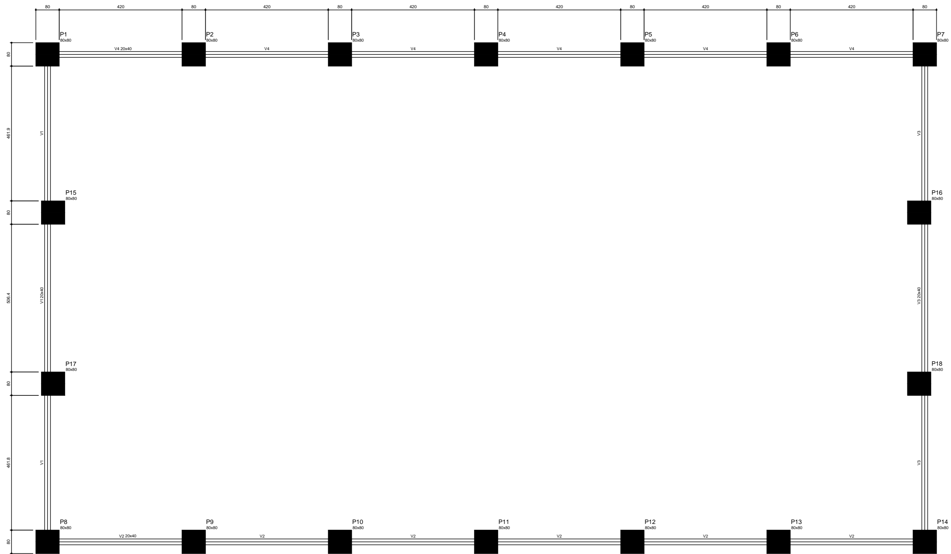
Forma do pavimento Baldrame escala 1:50
